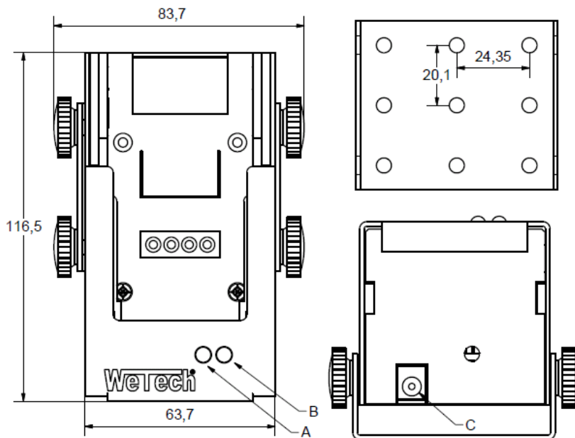
Schemazeichnung WTC689
